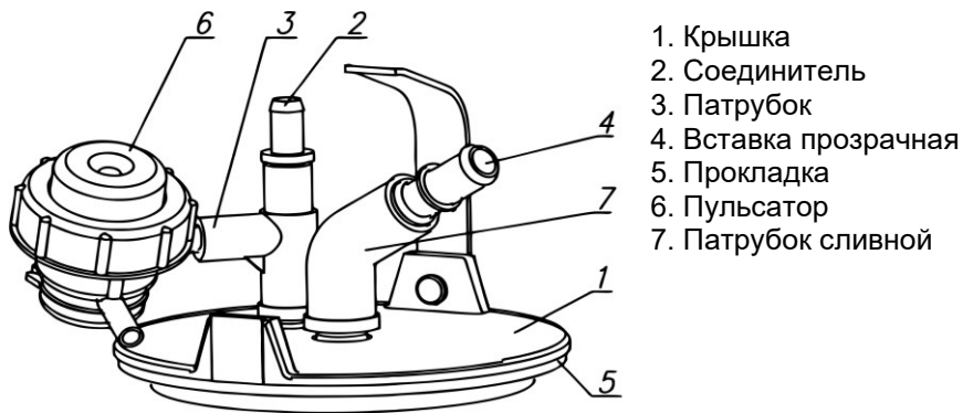
Рис. 5 Крышка ведра в сборе
